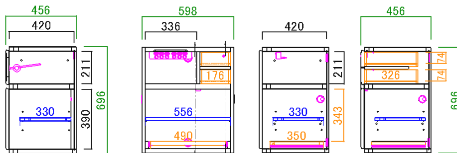
60家電 サイズ：W598 D456 H696
