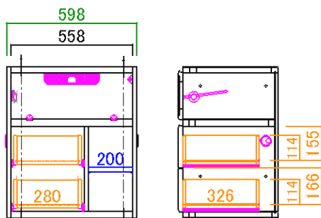
60AV サイズ：W598 D456 H696
