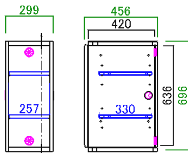
30板扉L 30板扉R サイズ：W299 D456 H696
