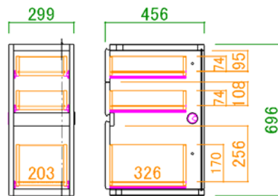
30引出 サイズ：W299 D456 H696
