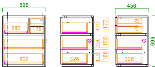
60引出 サイズ：W598 D456 H696
