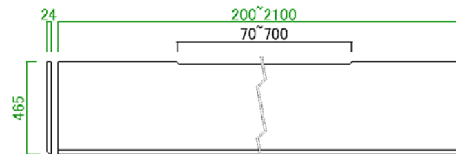
オーダー天板 D465 H24 サイズ：W200~900 サイズ：W910~1200 サイズ：W1210~1500 サイズ：W1510~1800 サイズ：W1810~2100
