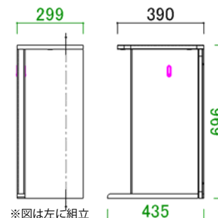
エンドパネル サイズ：W299 D435 H696
