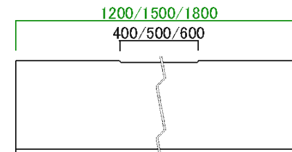
1200天板 サイズ：W1200 D465 H24 1500天板 サイズ：W1500 D465 H24 1800天板 サイズ：W1800 D465 H24
