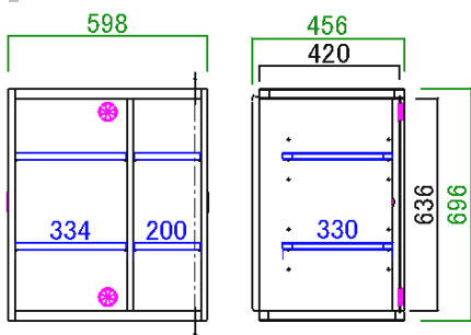
60板扉 サイズ：W598 D456 H696
