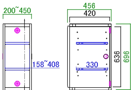
幅調整キャビネットL 幅調整キャビネットR サイズ：W200~450 D456 H696
